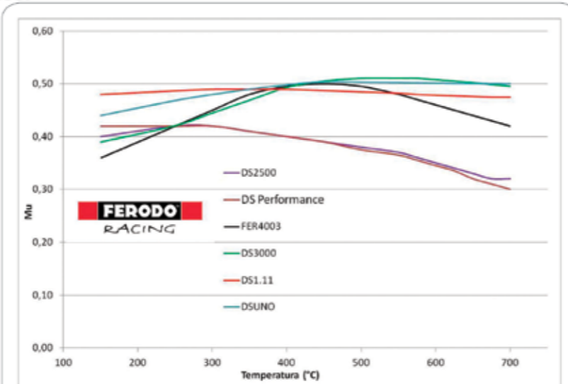
Il diagramma del banco prova dimostra che DS Performance ha una frenata iniziale ("bite") molto elevata e rimane sui stessi livelli di frenata come la DS2500 (pastiglia solo per uso Racing) fino a una temperatura di 600°C. Le pastiglie DS Performance è paragonabile alle DS2500 - ma con il grande vantaggio dell'omologazione stradale R90 per circolare sulle strade italiane.
